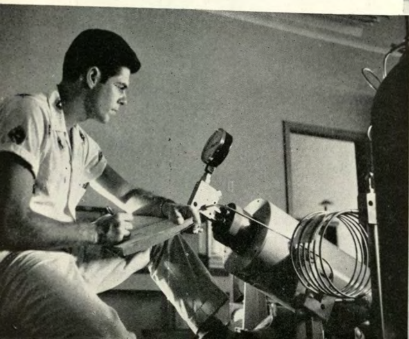
Experimentos de hidrogenación catalítica, realizados por Jorge Blasco para su tesis de grado.
